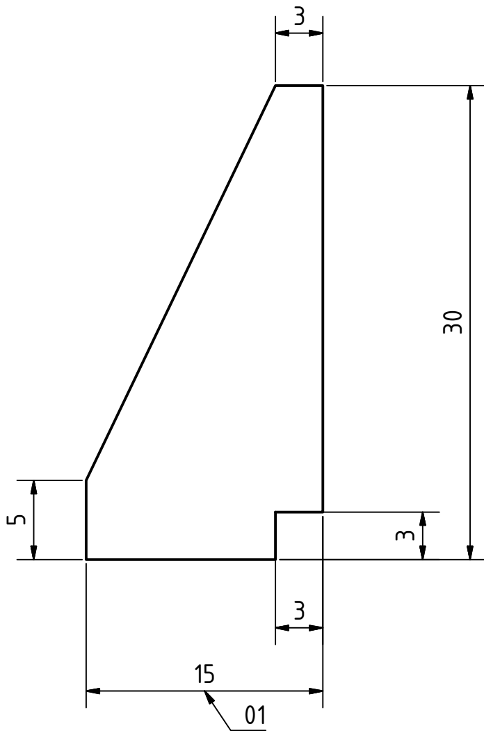
ANSICHT1 ( 2 : 1 )
