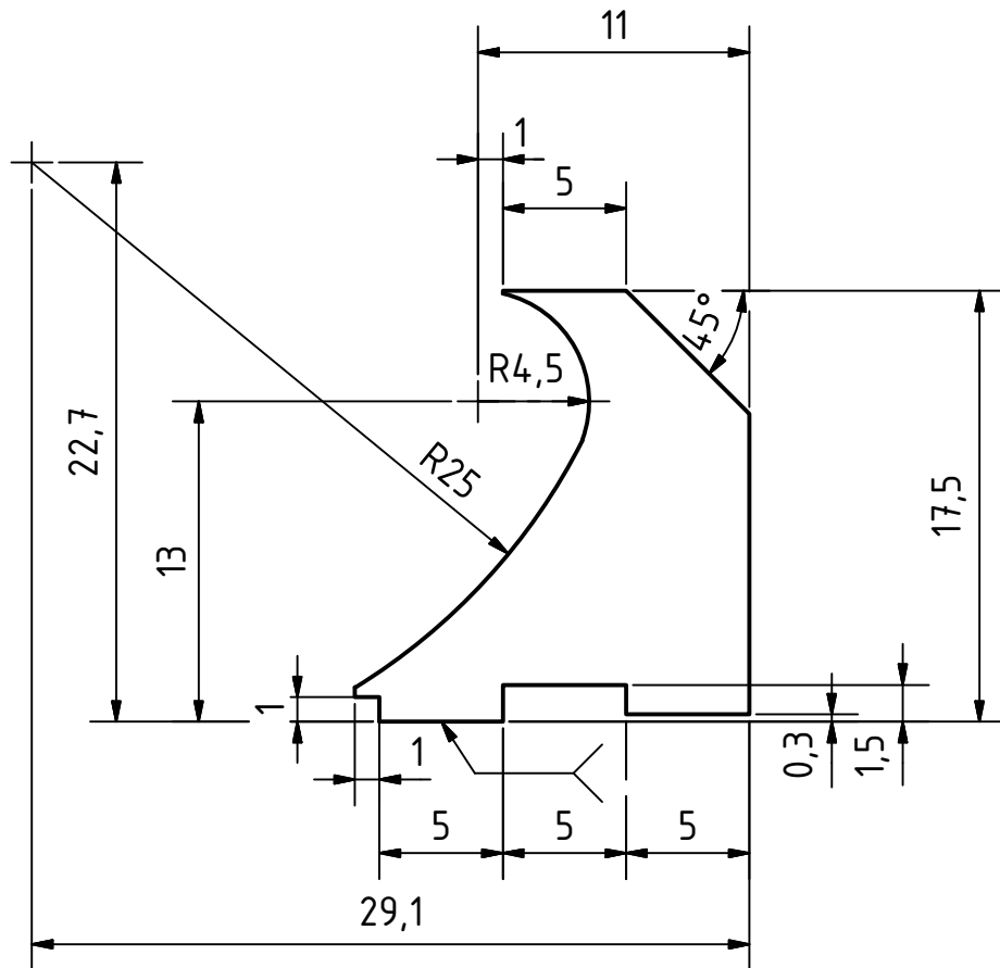
ANSICHT1 ( 2:1 )
