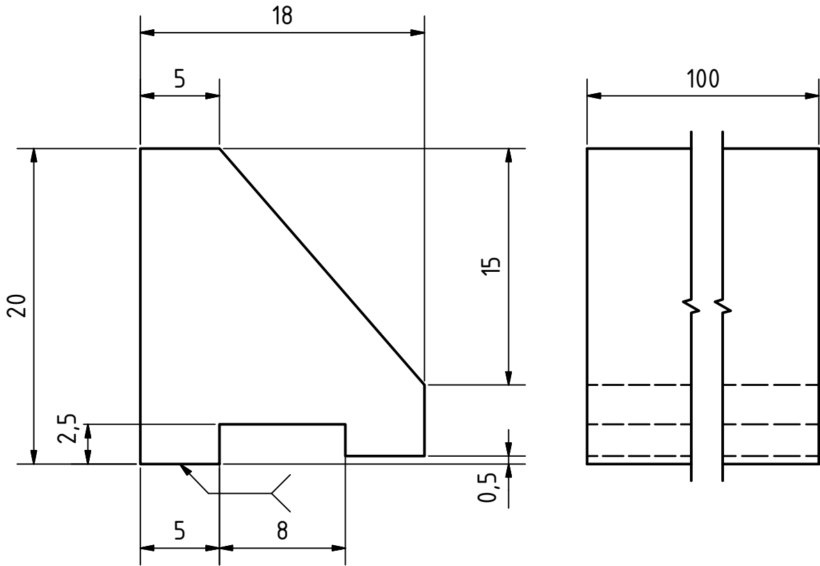
ANSICHT1 ( 2:1 )
