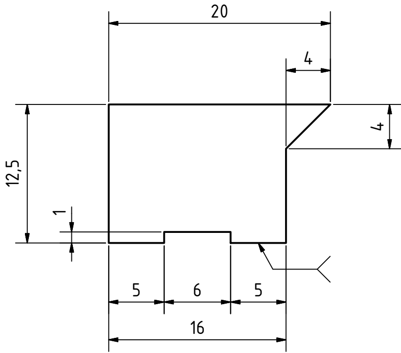
ANSICHT1 ( 2 : 1 )
